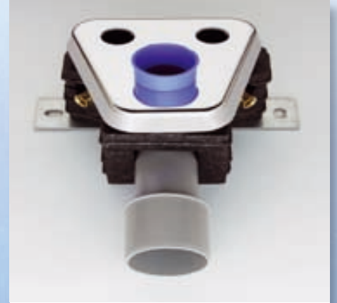
Монтажный узел PRINETO .
